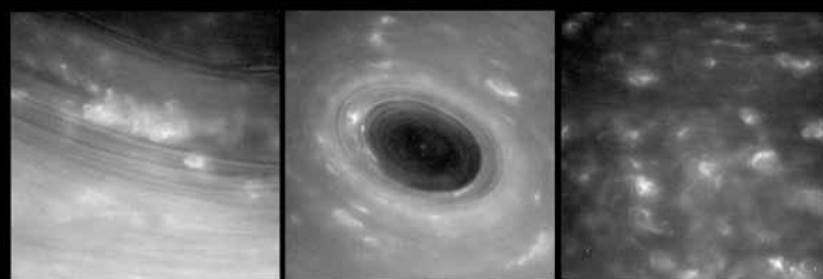
FIGURA 2: AS PRIMEIRAS IMAGENS DE SATÚRNO, AINDA SEM PROCESSAMENTO, OBTIDAS NO PRIMEIRO "MERGULHO" DA CASSINI.
