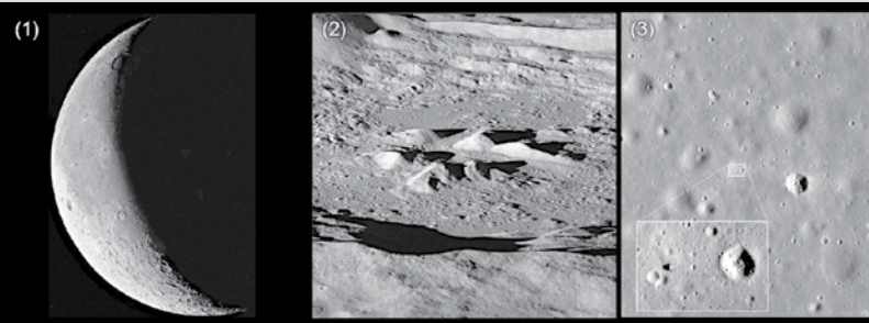
(1) A LUA VISTA DA TERRA, PELO OBSERVATÓRIO EUROPEU DO SUL. (2) OS MONTES NO CENTRO DA CRATERA HAYN COM UMA ALTURA DE 1,5 KM. (3) O LOCAL ONDE A APOLO 11 ALISNOU, ONDE O PEQUENO ROBOTICISTA MOSTRA O MÓDULO LUNAR E O RASTRO DEIXADO PELOS ASTRONAUTAS NA SUPERFÍCIE. CRÉDITOS DAS IMAGENS: OBSERVATÓRIO EUROPEU DO SUL E NASA - LUNAR RECONNAISSANCE ORBITER.
