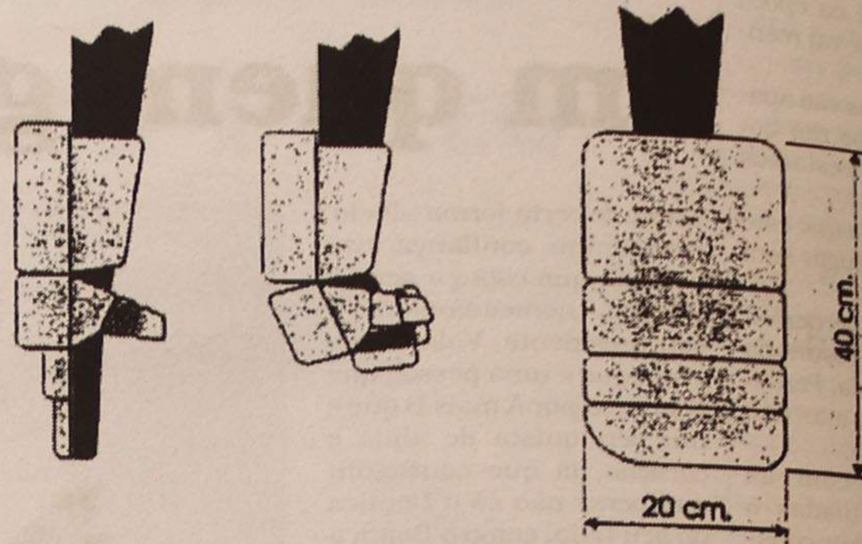
Luvas de guarda-redes - medidas máximas permitidas
