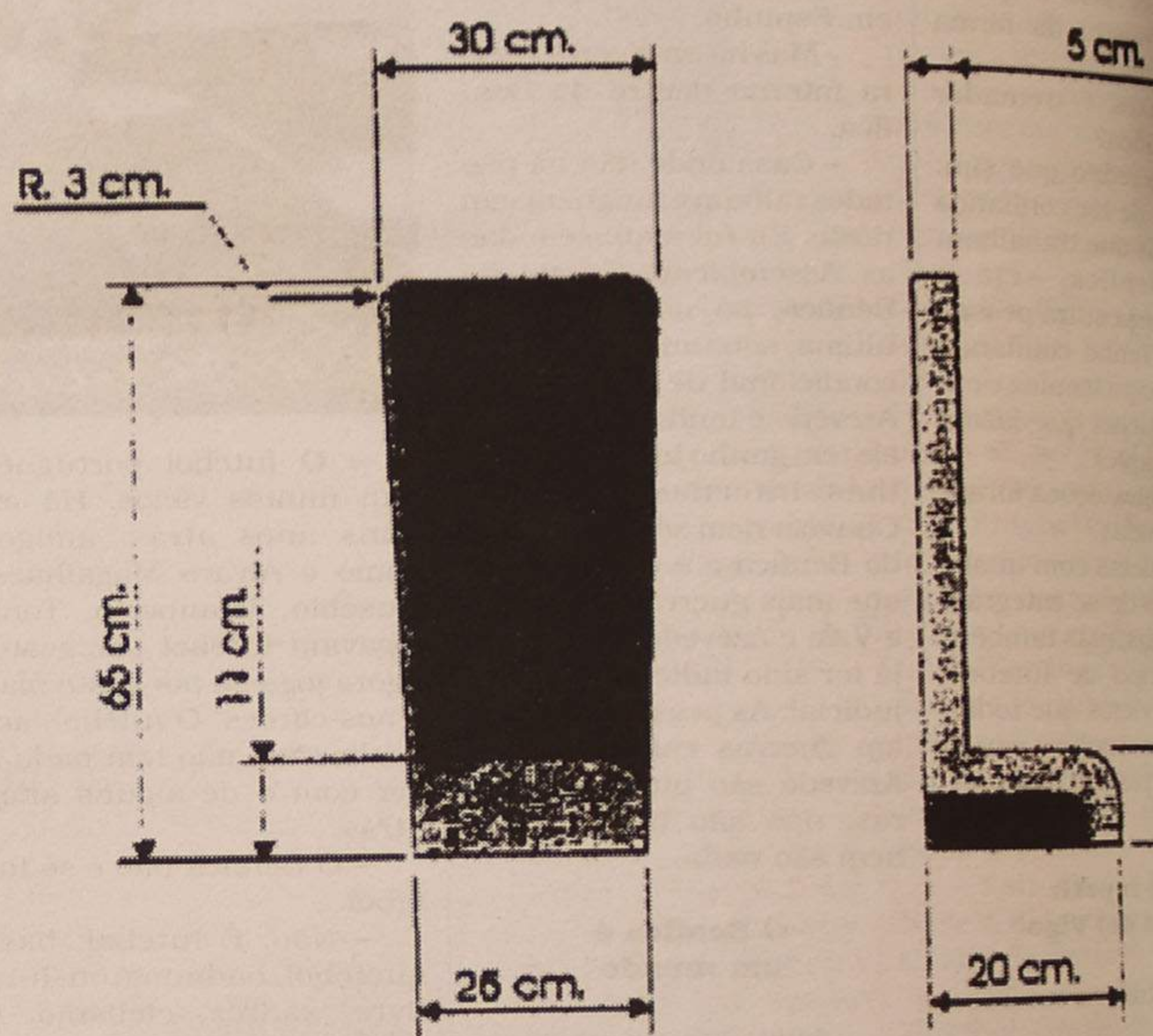
Caneleiras de guarda-redes - medidas máximas permitidas
